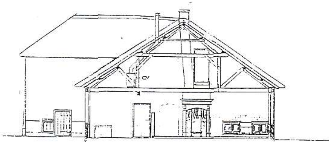
Doorsnede tussendeel (nieuw)
